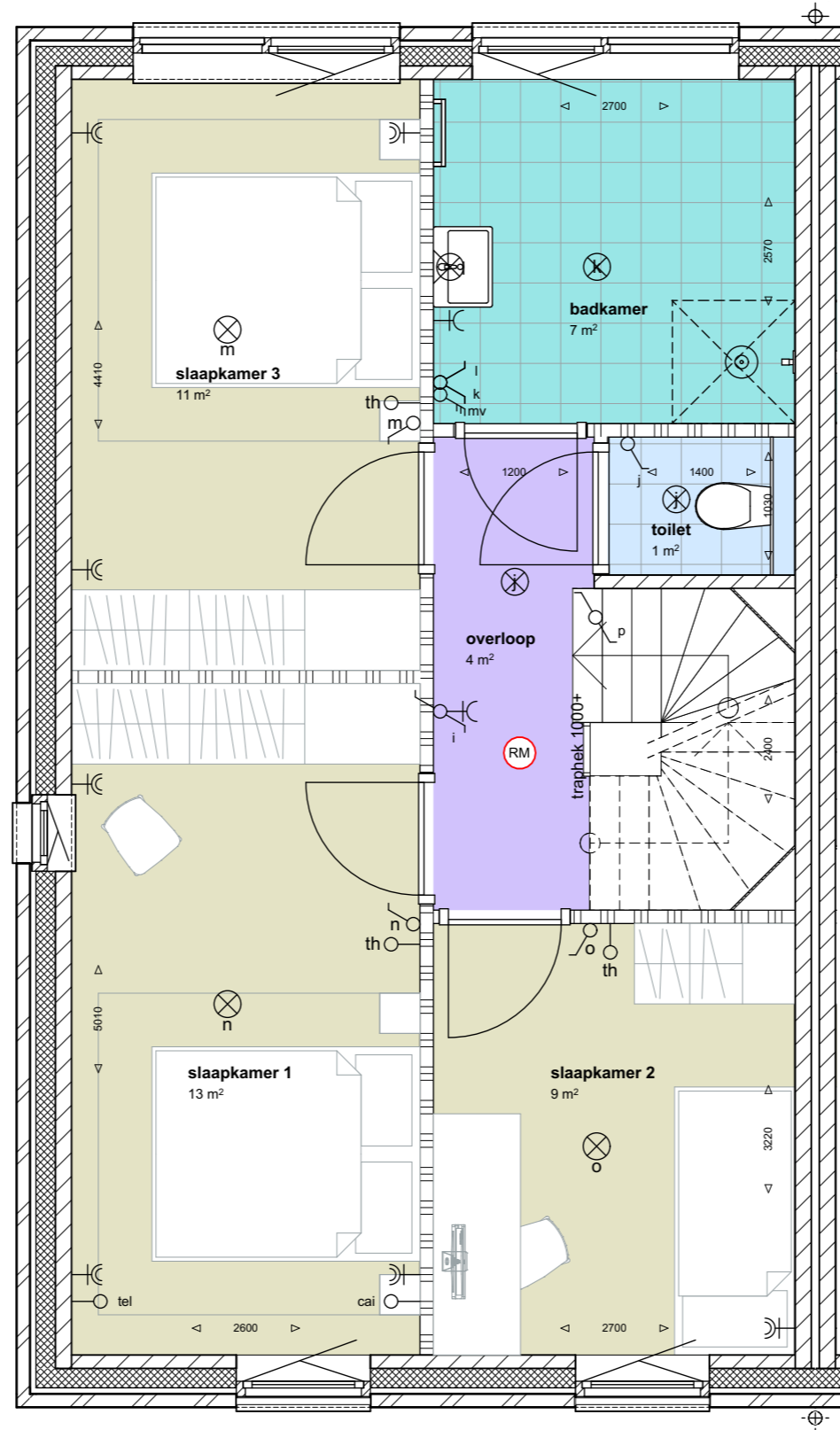
1e verdieping
