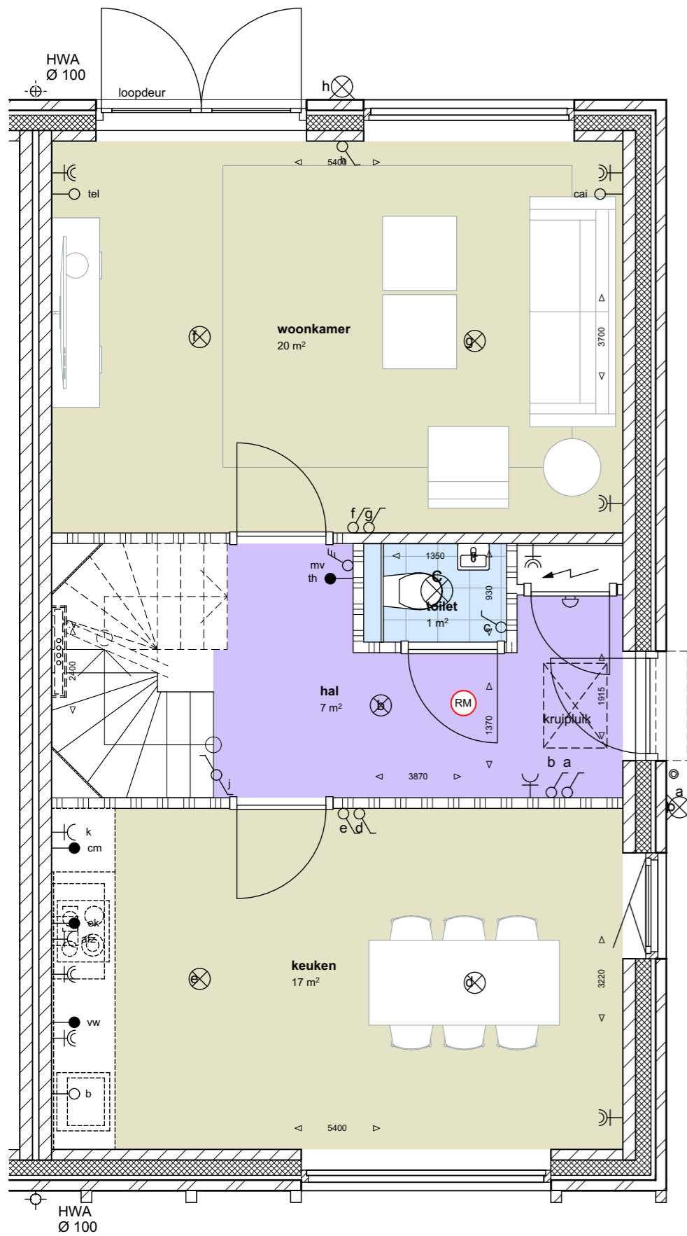
begane grond
