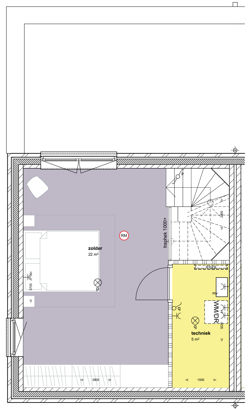
2e verdieping
