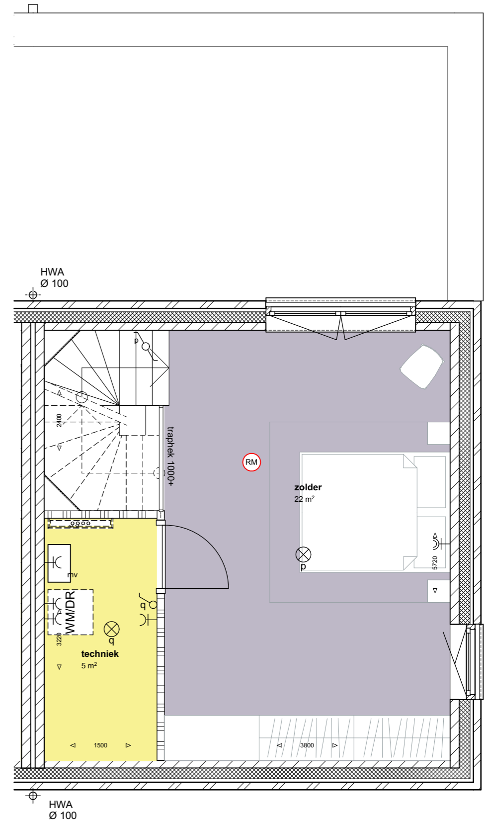
2e verdieping
