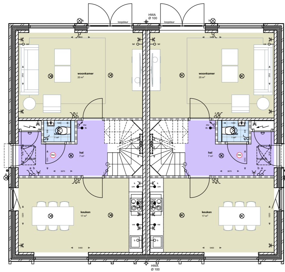
begane grond
