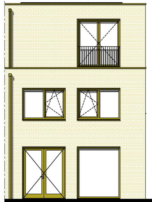
achtergevel
