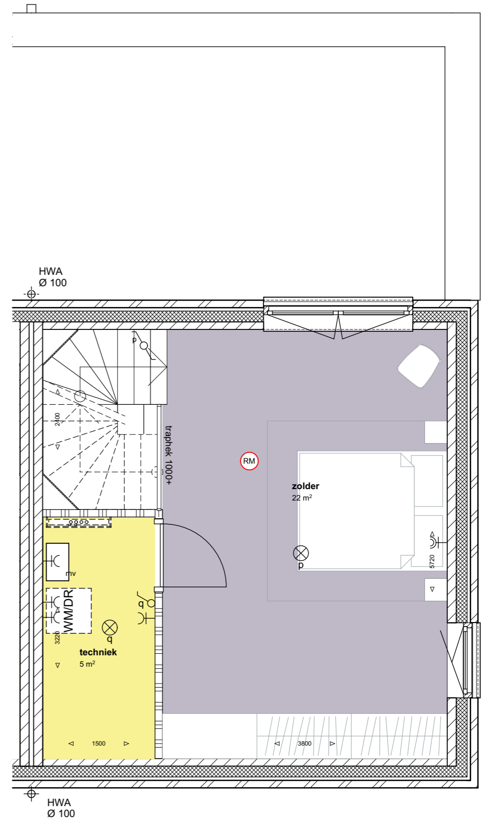
2e verdieping
