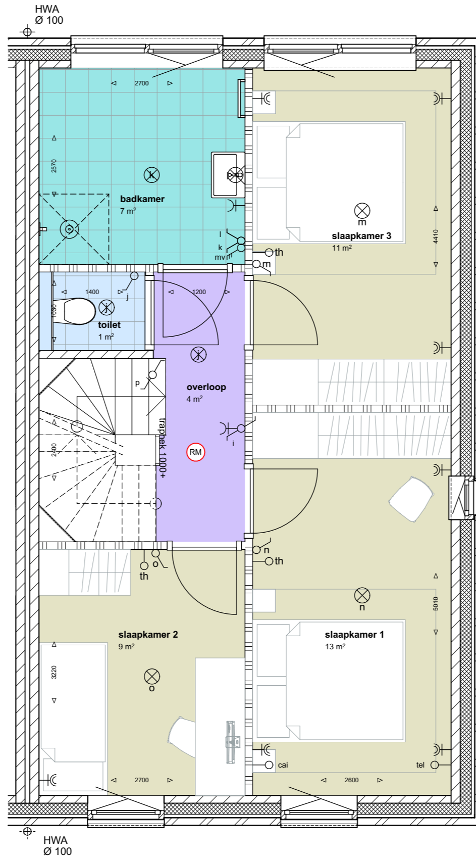
1e verdieping
