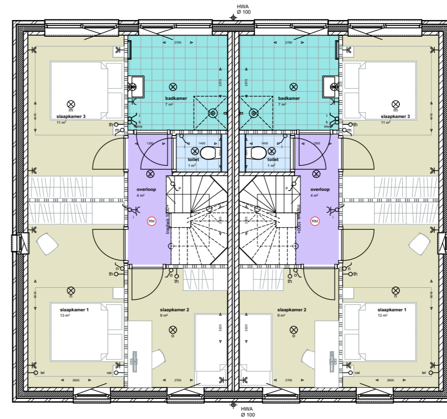
1e verdieping
