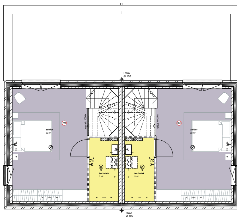
2e verdieping
